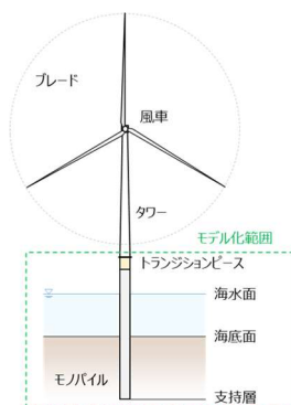
図 1.3.2b-7 地震力を考慮した洋上風車応答解析モデル
