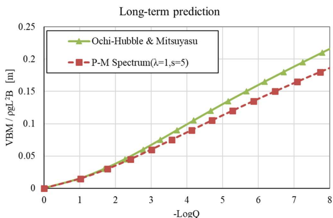
図 1.2.165 波スペクトルモデルによる長期分布の比較
