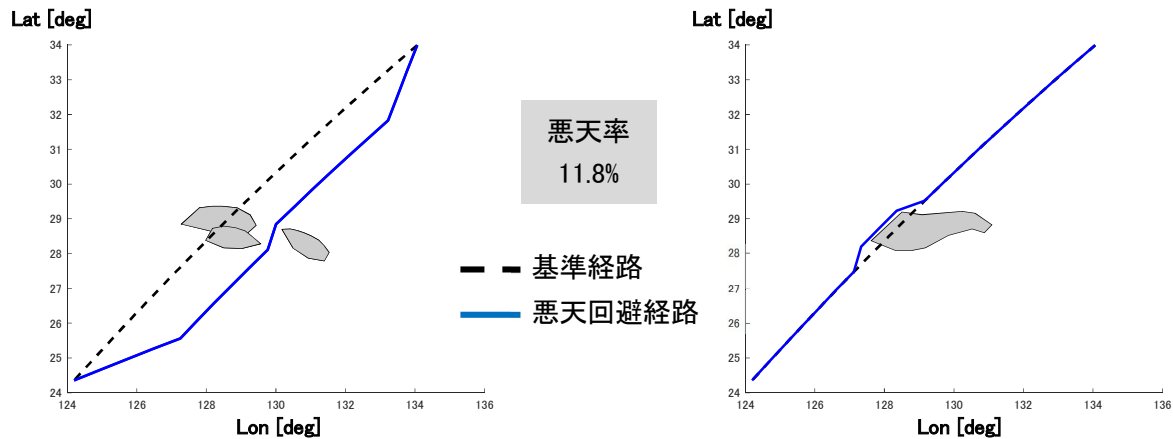
図 1.4.22 悪天回避経路の生成結果
