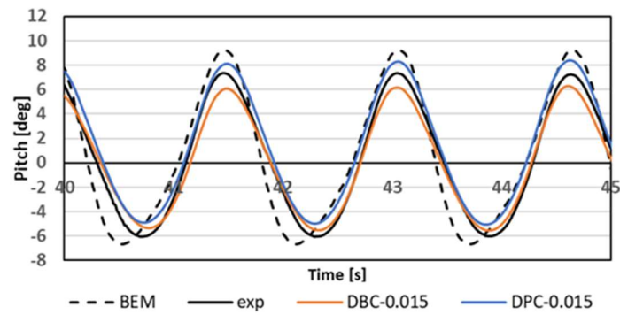
図 1.2.7 粒子法を用いた大波高船体運動(Pitch)の計算結果
