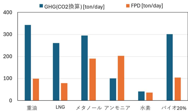
図 1.2.78 1日当たりの燃料消費量及び GHG 排出量
