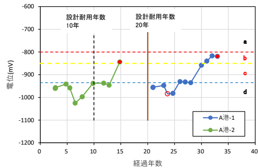
図 1.3.3b-2 鋼構造物の電気防食の劣化度判定の見直し(案)及び定期点検結果の一例
