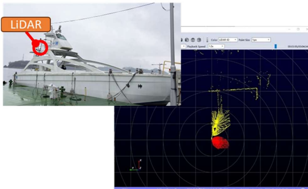
図 1.2.66 LiDAR 計測
