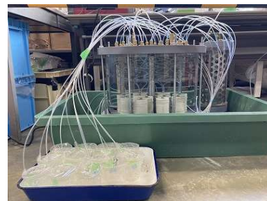
(b) 改良した劣化促進試験機
