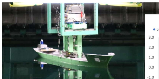
図 1.2.49 内航タンカー模型 の操縦流体力の計測
