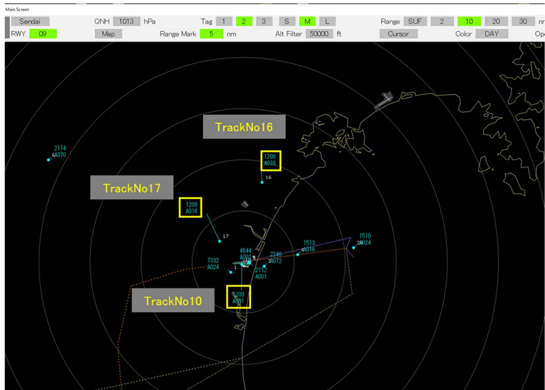
図 1.4.43 モード A/C 対応 MLAT による F/B 機 の分離・識別の結果
