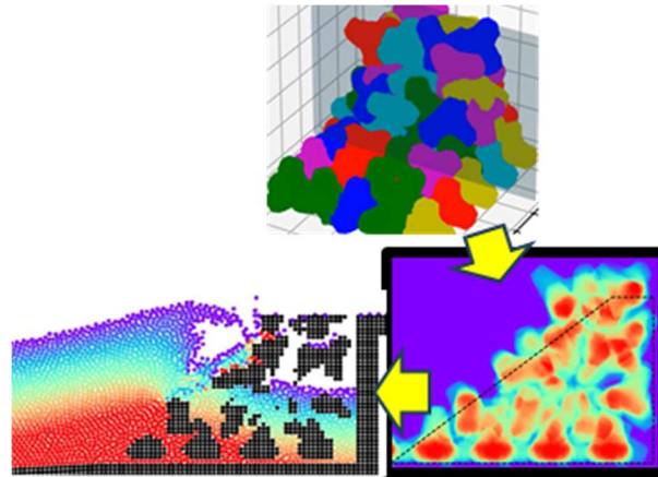
図 1.3.1b-2 ブロックの3次元幾何特性を反映した2次元モデル
