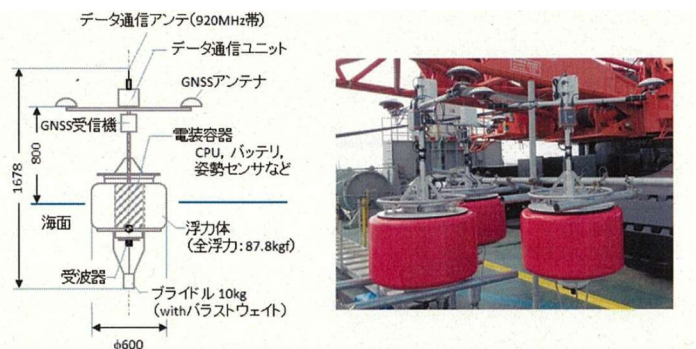
図 1.3.4a-4 浮上局概要図
