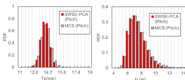
図 1.2.166 実船データを用いた手法の検証結果 (主成分分析手法 SWSE-PCE とモンテカルロシミュレーション法による確率密度の比較)
