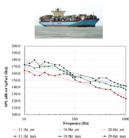
図 1.2.83 コンテナ船を対象とした簡易推定法と実船計測結果の比較
