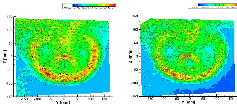
図 1.2.72 SWBC 船型のプロペラ面の主流方向流速の標準偏差(左:スタッド無し、右:スタッド有り)(7.2knot)
