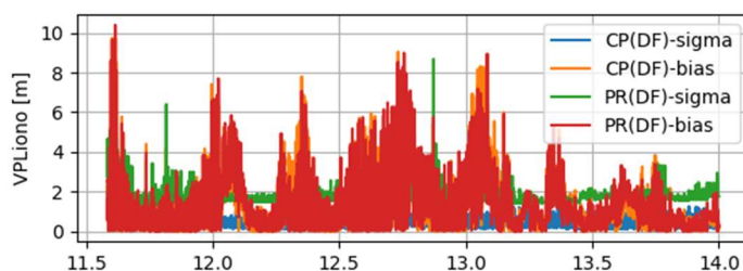
図 1.4.1 雷離圏擾乱時の DFMC GBAS 雷離圏モニタの検証
