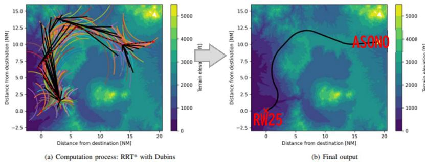
図 1.4.49 Dubins パスを用いた経路計算の途中 図 1.4.50:生成した経路のひとつ
