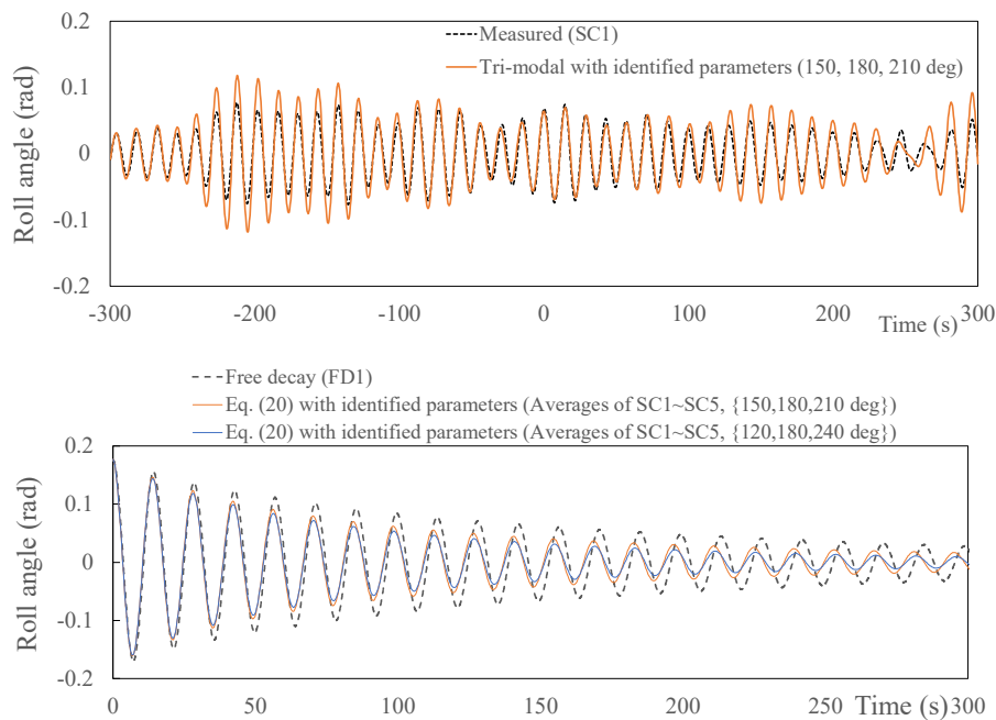
図 1.2.11 同定された減衰及び固有周期を用いた多方向不規則波中の横揺れの再現結果(上)及び自由横揺れの再現結果(下)
